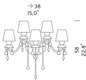
672/A3+2 5 x MAX 42W E14
